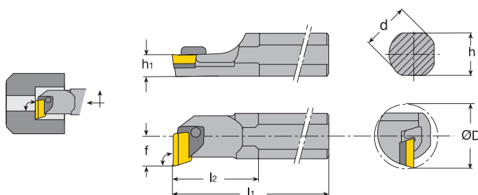
Bild zeigt rechte Bohrstange, linke Bohrstange spiegelbildlich
